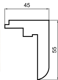
Übergangleisten für Dehnungsfugen
