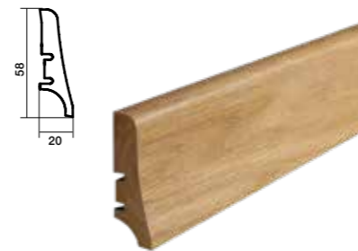
Sockelleiste Eiche lackiert P20 – P2001011A
