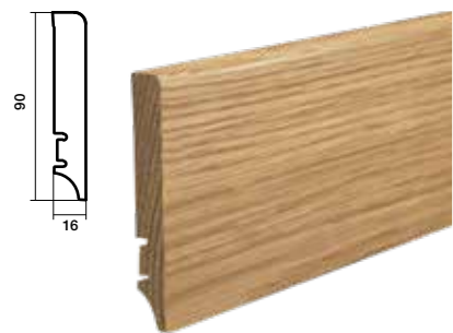
Sockelleiste Eiche lackiert P61 – P6101011A
